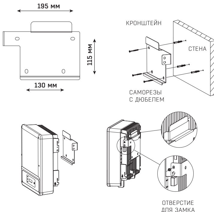
Рисунок 3.4.4 Инструкция по креплению инвертора на поверхность
